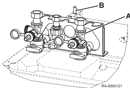
Fig.14 Fixer le kit vanne d'arrêt AEH (accessoire)
