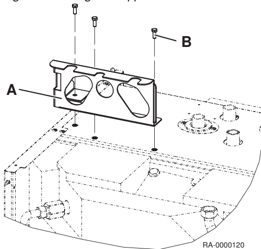
Fig.14 Fixer le kit vanne d'arrêt AEH (accessoire)
