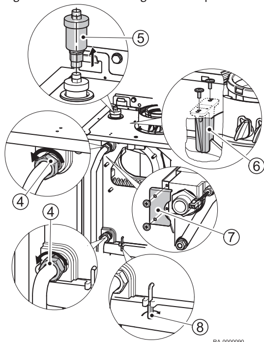
Fig.42 Retrait de l'échangeur thermique
