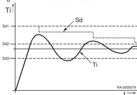
Fig.35 Différence de commutation
