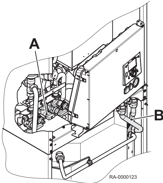
Fig.17 Raccordements hydrauliques chaudière-ballon / réseau
